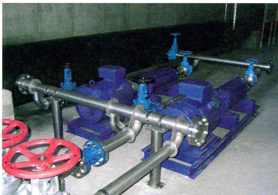
particolare allacciamento pompa di sollevamento in località Spino al tubo di aduzione della sorgente.
